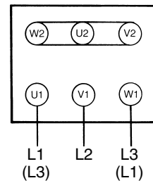
Couplage Y (tension haute)
