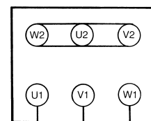
Y-kobling (høyspenning)
