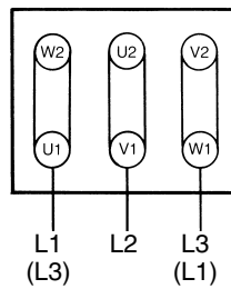
Couplage \Delta (tension basse)
