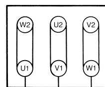
Δ-kobling (lavspenning)
