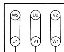
\Delta -koppling (lägre spänning)
