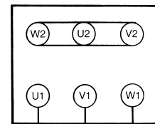
L1 L2 L3 (L3) (L1) \Upsilon -Schaltung (hohe Spannung)
