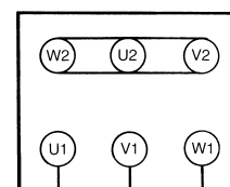
\Upsilon -koppling (högre spänning)
