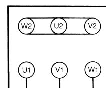
Circuito \Upsilon (alta tensione)
