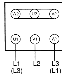
Połączenie w gwiazdę (wysokie napięcie)
