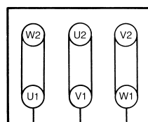
L1 (L3) L2 L3 (L1) Ligação- \Delta (Baixa corrente)
