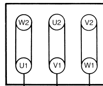
Conexión de triángulo (baja tensión)
