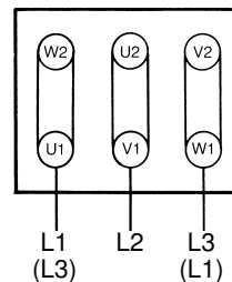
Połączenie w trójkąt (niskie napięcie)
