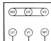
L1 (L3) L2 L3 (L1) Ligação \Upsilon (Baixa corrente)
