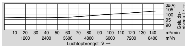
Δ schakeling (lage spanning)
